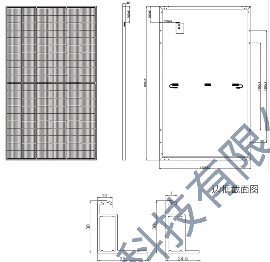
尺寸图纸 (mm)
